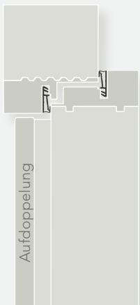
Schallschutzaufdoppelung bei Rubner KlimaHausTüren
